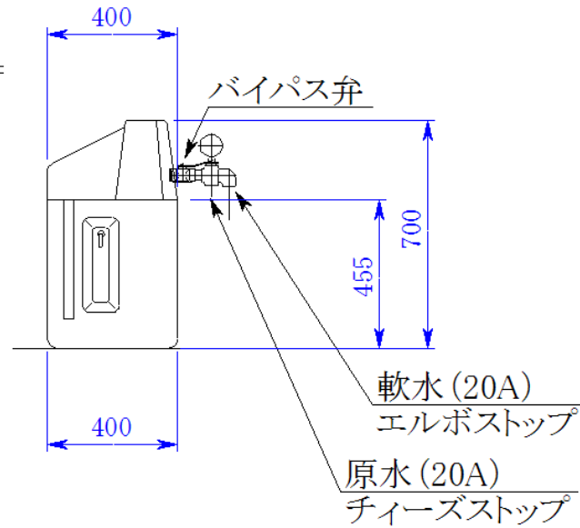
右側面図
